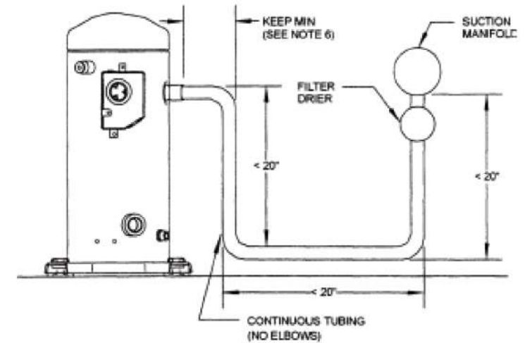
Figura 3 Disposiciones típicas de la línea de succión
