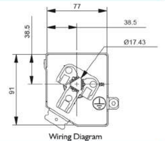
Figura 4 Conexiones de los terminales del motor
